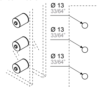
ART. 2AT.KIT.9906 25 mm 2AT.KIT.9908 30 mm 2AT.KIT.9910 35 mm
