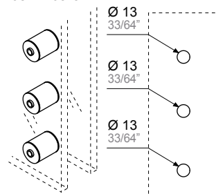
ART. 2CC.KIT.0006 25 mm 2CC.KIT.0008 30 mm 2CC.KIT.0010 35 mm
