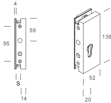
PLACCA CON SERRATURA SENZA MANIGLIA - CASE WITH LOCK WITHOUT LEVER HANDLE - PLAQUE AVEC SERRURES ANSPOIGNÉE - TÜRSCHILDMITSCHLIESSSYSTEM OHNE TÜRDRÜCKER
