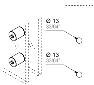
ART. 2AT.KIT.9905 25 mm 2AT.KIT.9907 30 mm 2AT.KIT.9909 35 mm
