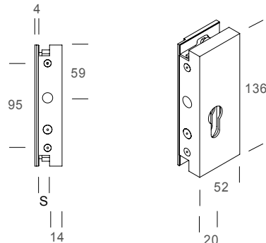
PLACCA CON SERRATURA SENZA MANIGLIA - CASE WITH LOCK WITHOUT LEVER HANDLE - PLAQUE AVEC SERRURES ANSPOIGNÉE - TÜRSCHILDMITSCHLIESSSYSTEM OHNE TÜRDRÜCKER
