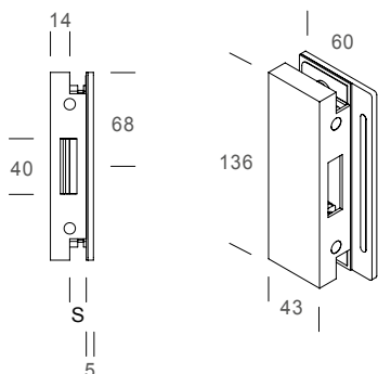
INCONTRO PER VETRO - STRIKE BOX - GÂCHE POUR VERRE - VERBINDUNG GLAS/GLAS
