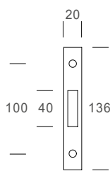
INCONTRO PER PROFILO - STRIKE PLATE - GÂCHE POUR PROFIL - PROFILVERBINDUNG
